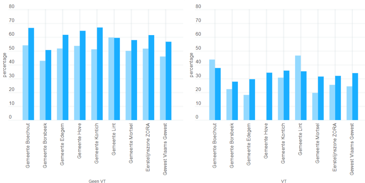
Grafiek 13 - Preventieve mondzorg 5-14 jaar; % met minstens 2 preventieve contacten met de tandarts in 2 verschillende jaren binnen een periode van 3 kalenderjaren (2012 vs. 2022 en geen VT vs. VT)
