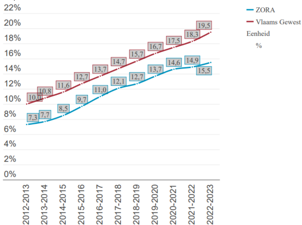
Grafiek 12 – evolutie leerlingen secundair onderwijs met thuistaal niet-Nederlands naar woonplaats, t.o.v. lln. SO, 2013-2023
