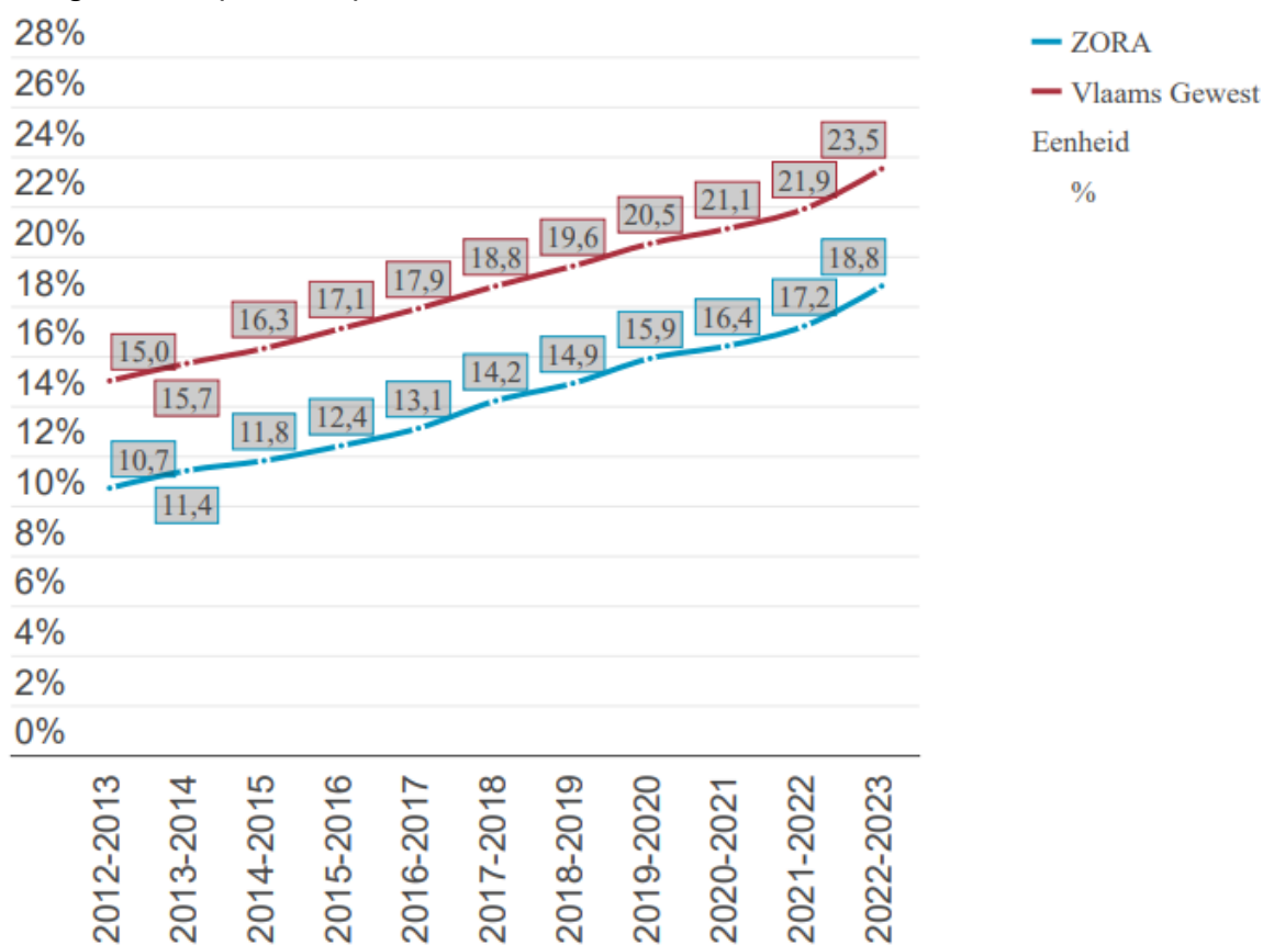
Grafiek 11 – Evolutie leerlingen gewoon basisonderwijs met thuistaal niet-Nederlands naar woonplaats, % t.o.v. lln. gewoon BO (2013-2023)
