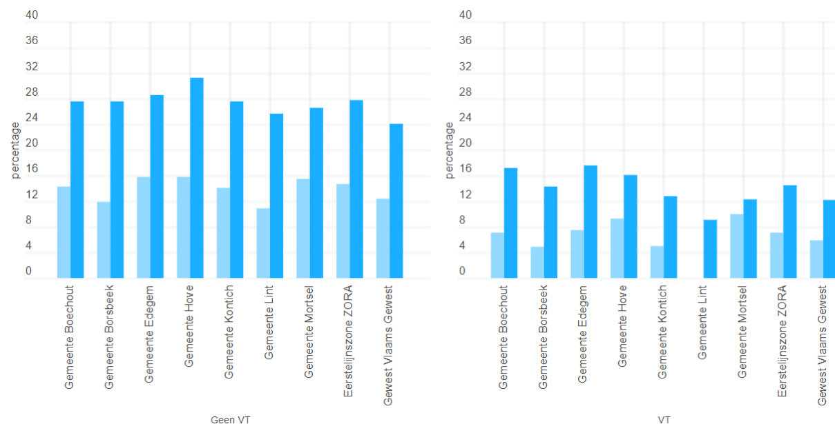
Grafiek 14 - Preventieve mondzorg 75+ jaar; % met minstens 2 preventieve contacten met de tandarts in 2 verschillende jaren binnen een periode van 3 kalenderjaren (2012 vs. 2022 en geen VT vs. VT)
