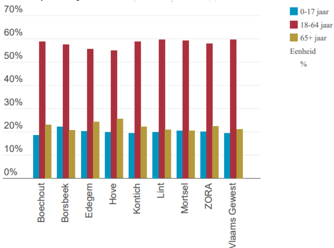
Grafiek 1 – leeftijdsverdeling in 2023
