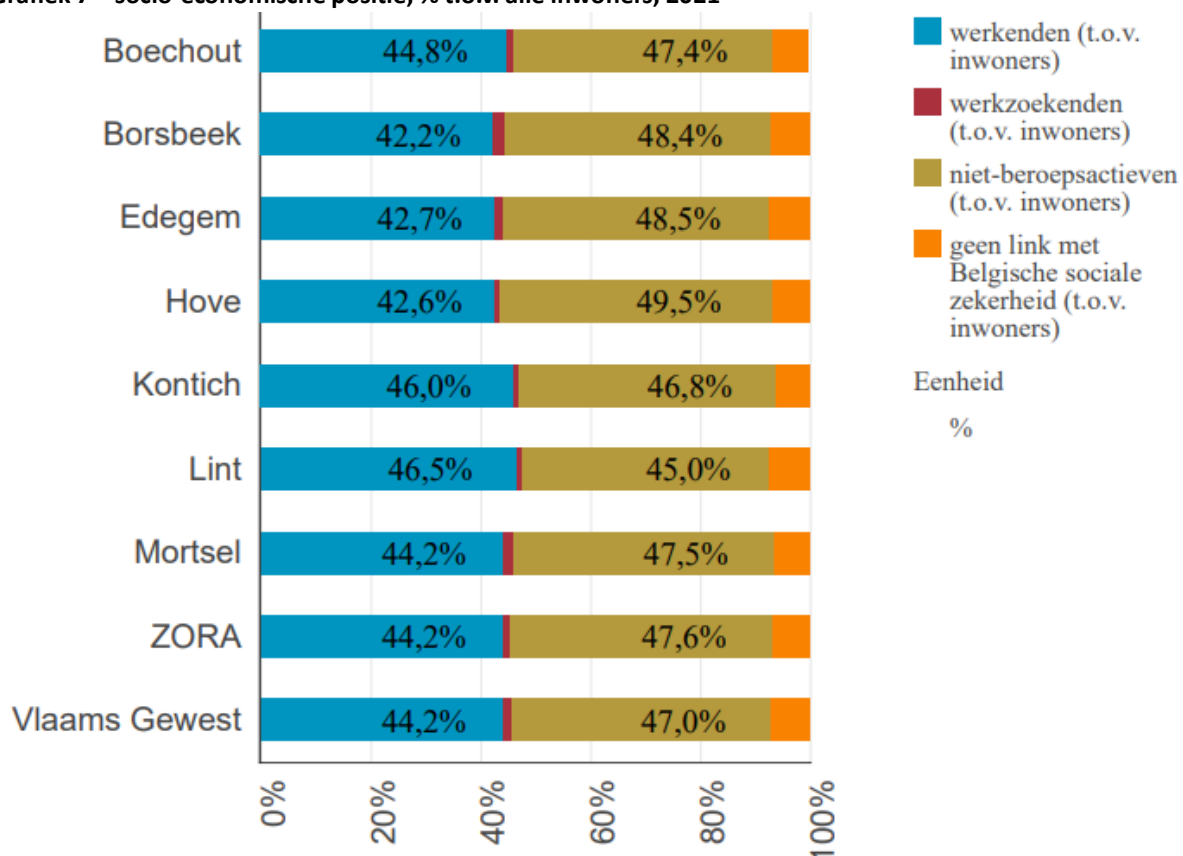
Grafiek 7 – socio-economische positie, % t.o.v. alle inwoners, 2021
