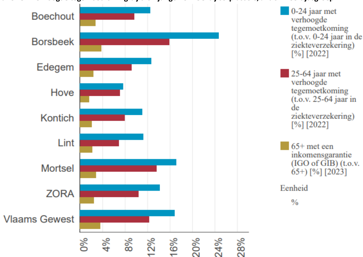
Grafiek 8 – verhoogde tegemoetkoming bij 0-64-jarigen en IGO bij 65-plussers, % t.o.v. leeftijdsgroep
