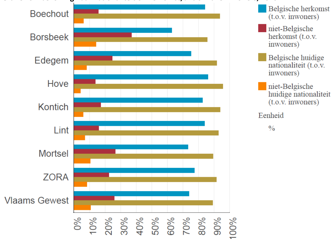
Grafiek 3 – bevolking naar nationaliteit en herkomst, % t.o.v. alle inwoners, 2023
