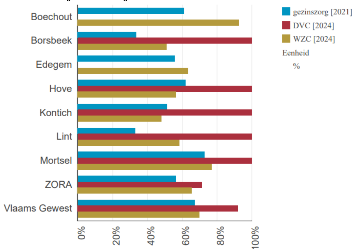
Grafiek 15 – realisatiegraad van het zorgaanbod voor ouderen
