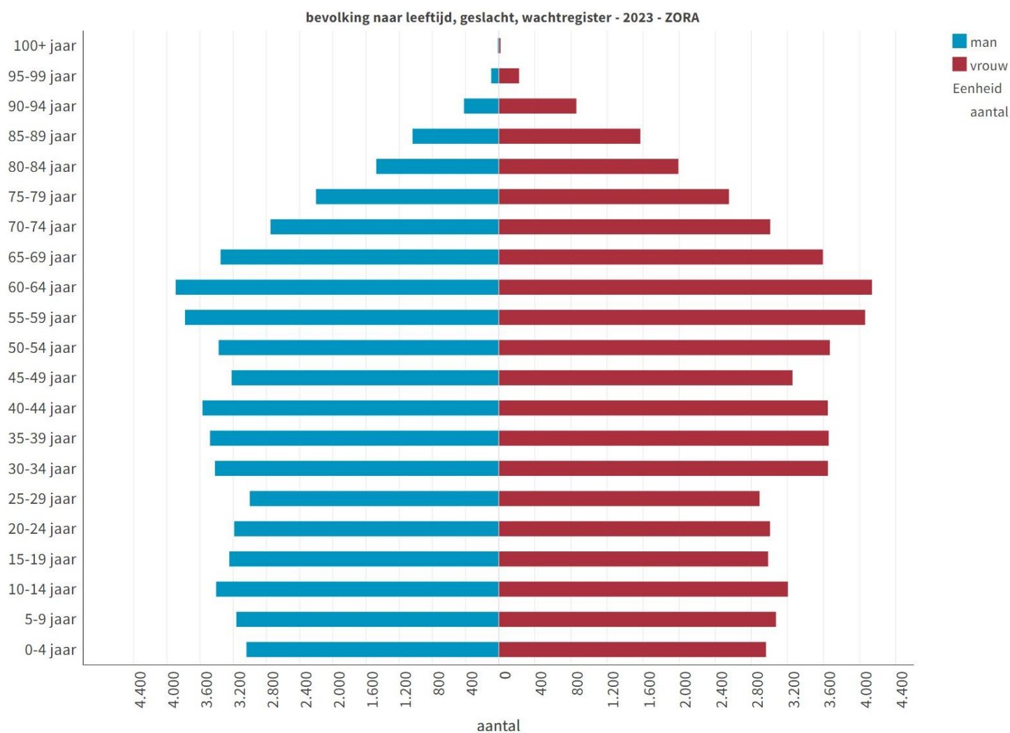
Grafiek 2 – bevolkingspiramide in 2023 (per leeftijdsklasse van 5 jaar)
