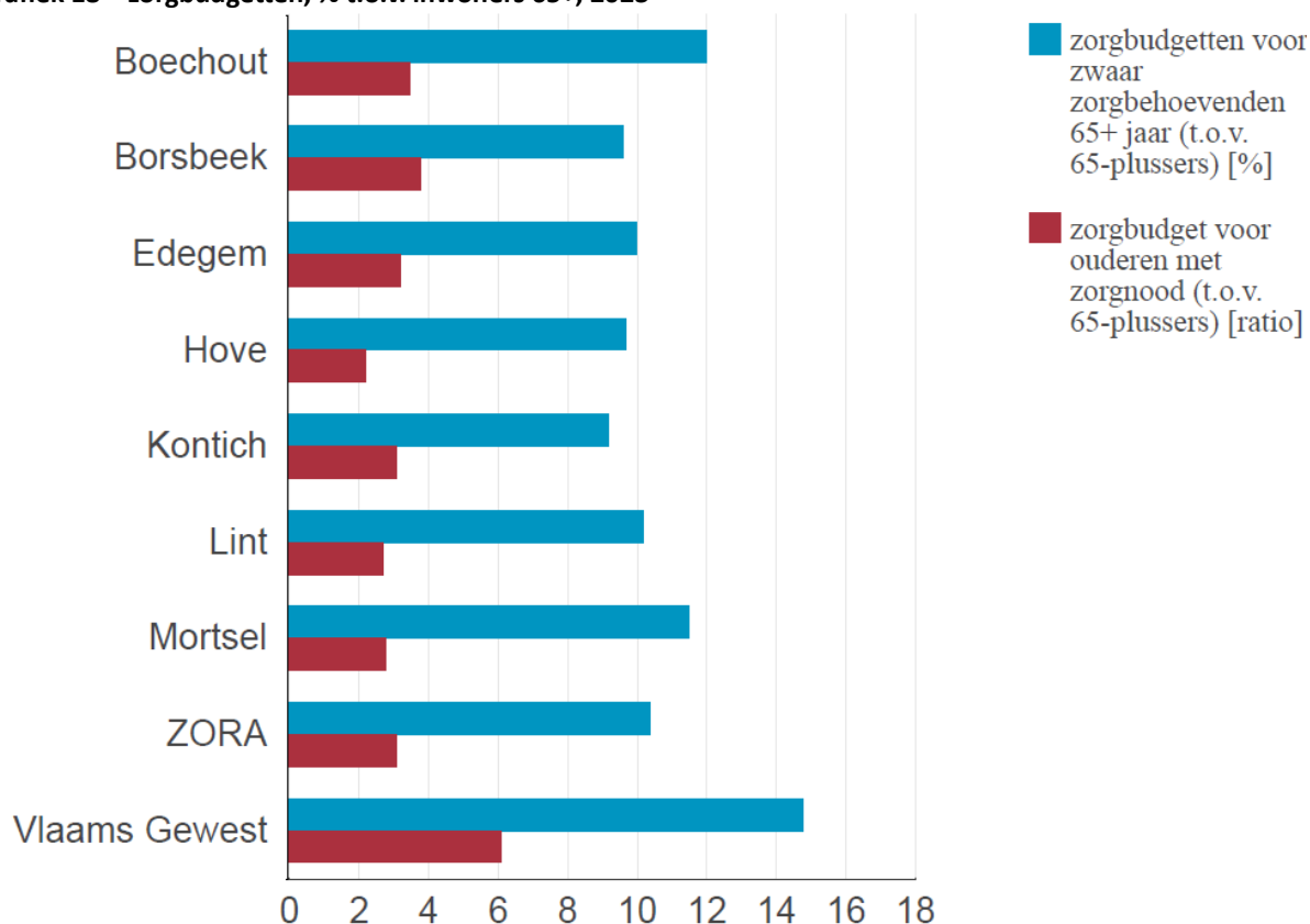
Grafiek 18 – zorgbudgetten, % t.o.v. inwoners 65+, 2023
