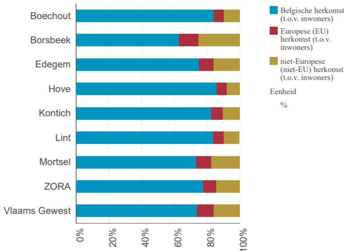
Grafiek 4 – Bevolking naar herkomst, opdeling EU- en niet-EU-herkomst, % t.o.v. alle inwoners, 2023
