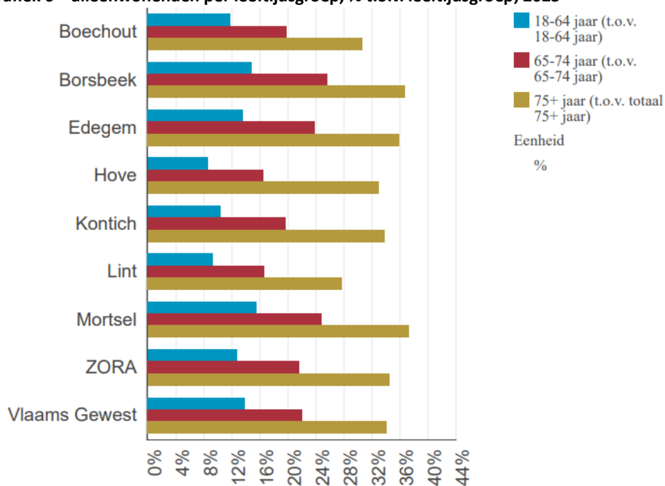
Grafiek 6 – alleenwonenden per leeftijdsgroep, % t.o.v. leeftijdsgroep, 2023
