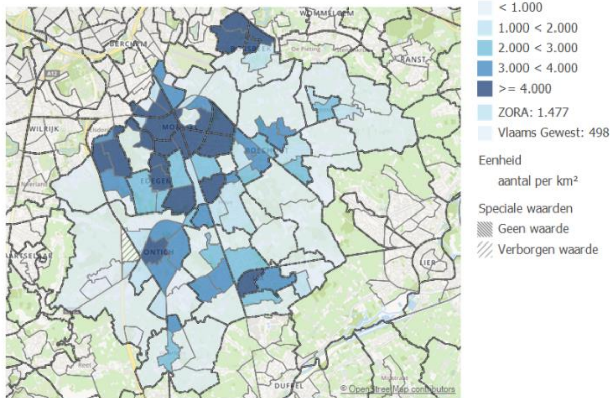
Kaart 1 - bevolkingsdichtheid op statistisch sectorniveau in 2023 ELZ ZORA.
