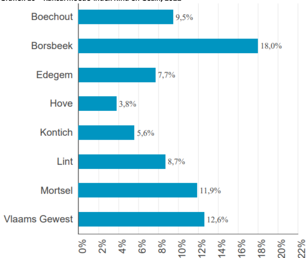
Grafiek 10 – Kansarmoede-index Kind en Gezin, 2022
